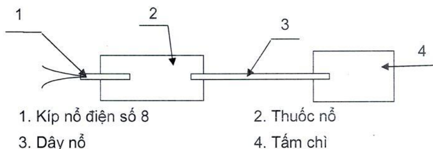
Hình 2 - Sơ đồ xác định khả năng chịu nước
