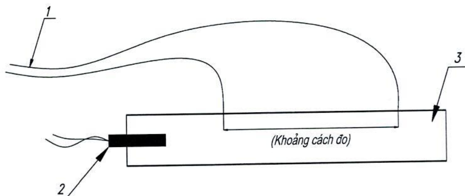
1. Dây quang 2. Kíp nổ điện số 8 3. Thuốc nổ Pentrit
